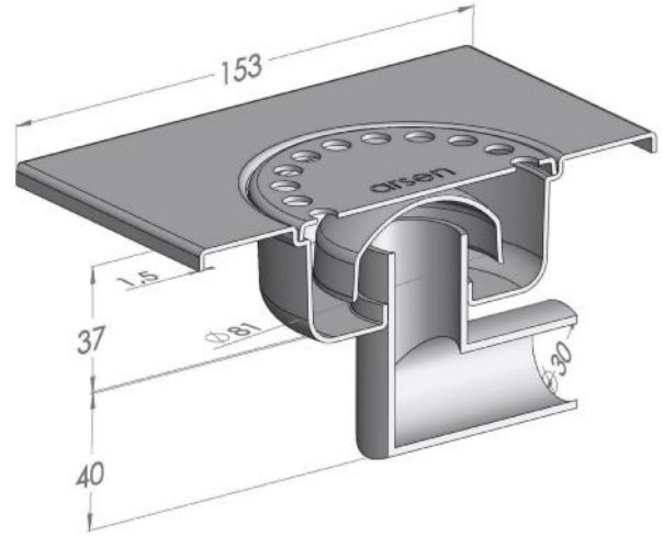
TİP/TYPE : 150YC30
