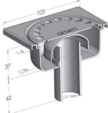
TİP/TYPE : 100AC30
