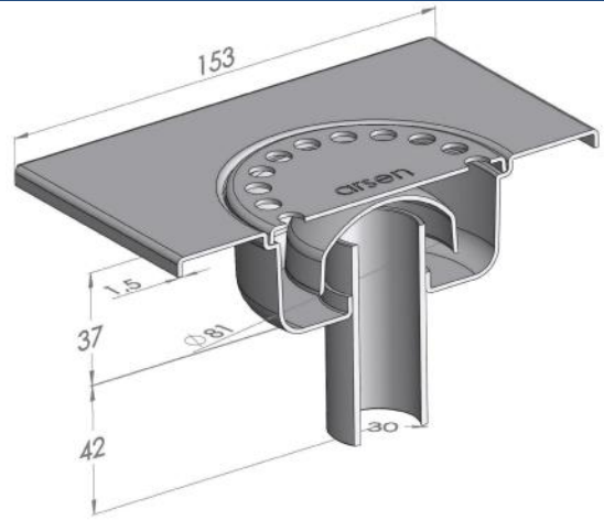
TİP/TYPE : 150AC30
