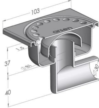
TİP/TYPE : 100YC30
