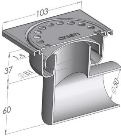
TİP/TYPE : 100YC50
