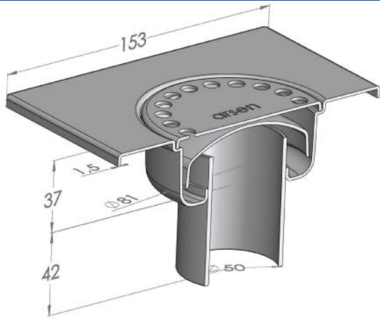
TİP/TYPE : 150AC50
