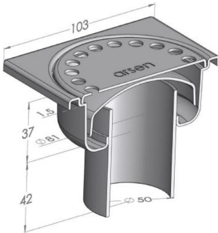
TİP/TYPE : 100AC50
