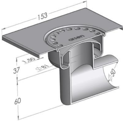
TİP/TYPE : 150YC50
